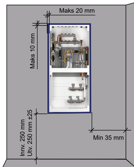
Installasjonsmål LK Kombiskap UNI-Xvs RAD.
