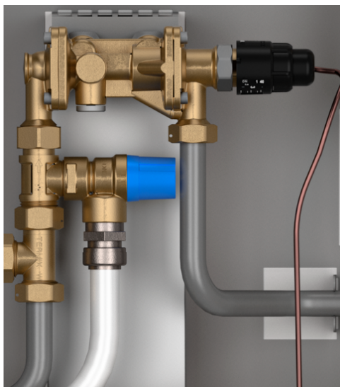
Varmeveksleren med tappevannsregulator.
