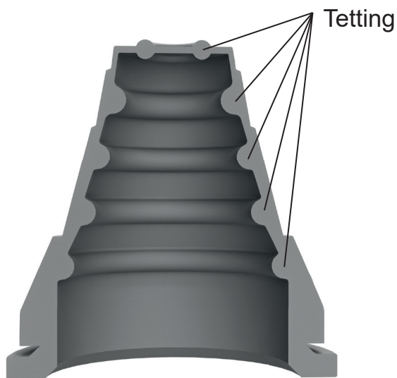
Tverrsnitt av rørgjennomføring som viser rørtettingens plassering.
