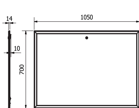
LK Ramme/luke GV 1050, UTV
