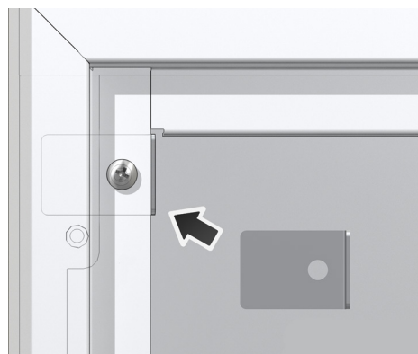
Blikkplate og skrue til LM Ramme/luke GV UTV.
