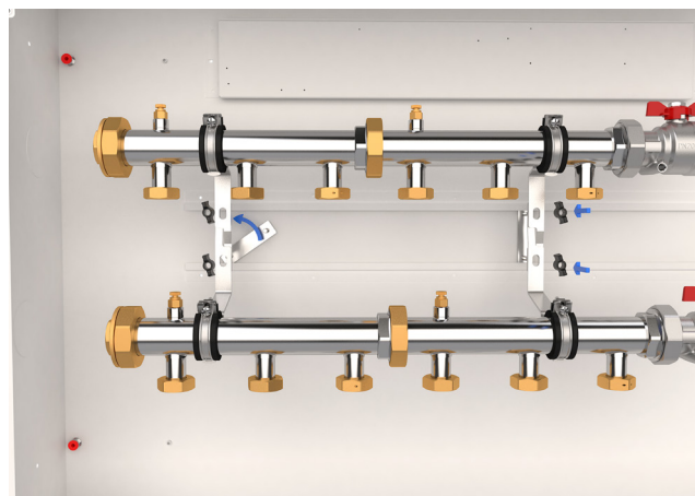
Montering av LK Fordeler Qmax G50.
