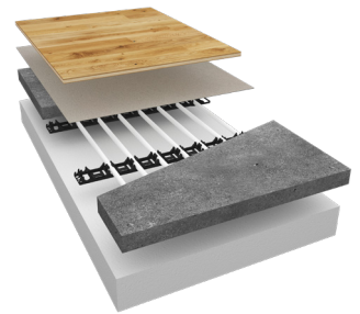
LK Leggeskinne Combi 16/20
