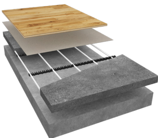
LK Leggeskinne Click 12
