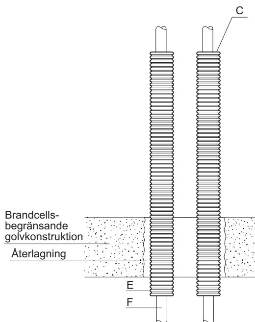
Rör genomgång genom brandcells-begränsande golv.
