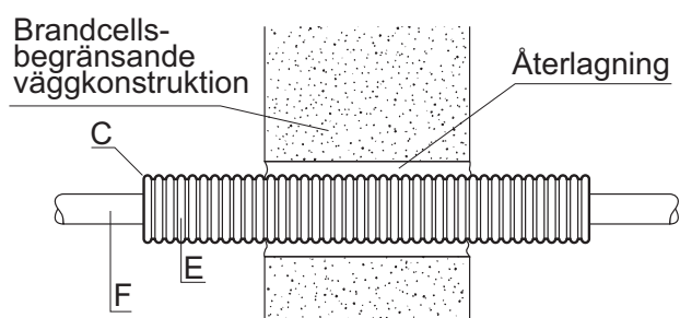
Rör genomgång genom brandcells-begränsande vägg.
