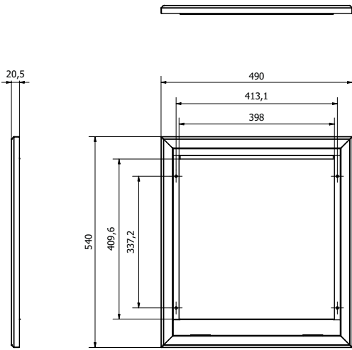
Förhöjningsram GV 450x500 LK Increased Frame UFH 450x500 LK Utforingsramme GV 450x500 LK Korotuskehys LL 450x500
