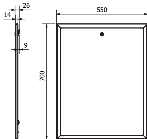
LK Ramme/luke GV 550, UTV
