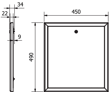
LK Ramme/luke M60n, UTV
