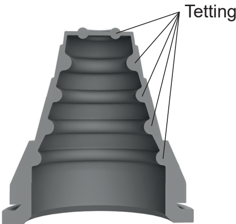
Plassering Tverrsnitt av rørgjennomføring viser rørtettingens plassering.
