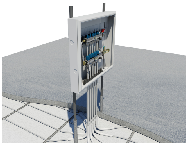
LK Skapstativ L2 med LK Fordelerskap
